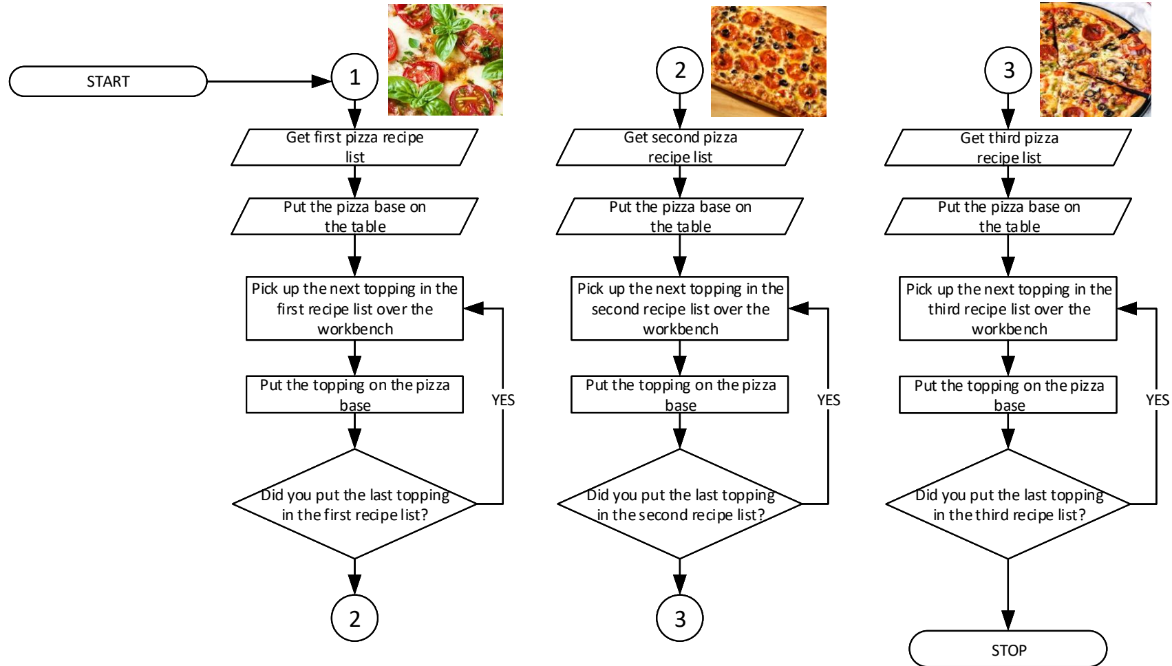
Diagramm 2 - Gemischter Algorithmus
