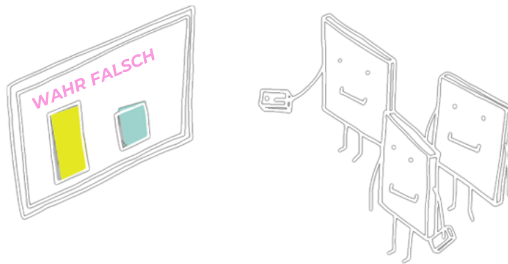
Abbildung 3 - Bewertung
