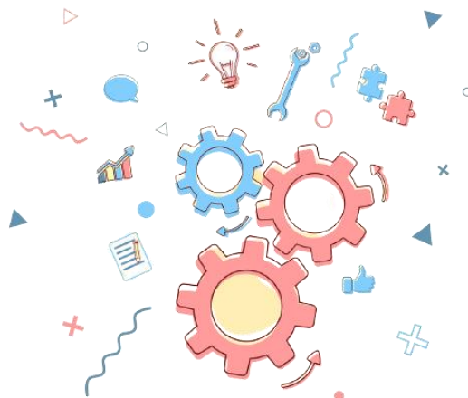
Abbildung 8 - Designprozess
