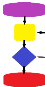
Abbildung 1 - Algorithmisches Denken
