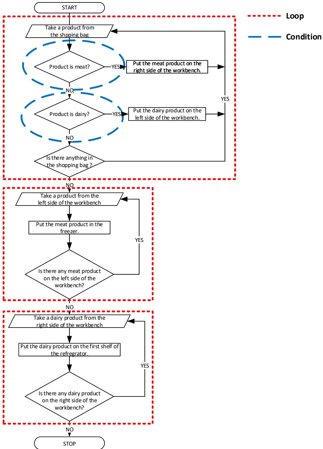
Diagramm 4 - Die Schleifen und Bedingungen im Flussdiagramm des neuen Algorithmus
