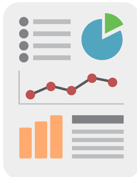
Abbildung 4 - Daten
